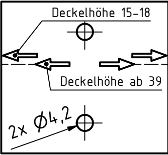
Bohrschablone (1 : 1)
