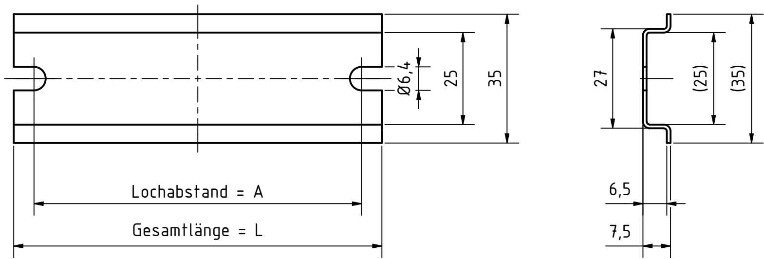
LÄNGEN DER TRAGSCHIENEN TS 35 x 7,5 --- PRODUKTGRUPPEN MBA, MBP, MBI
